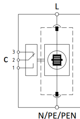
Принципиальная схема
