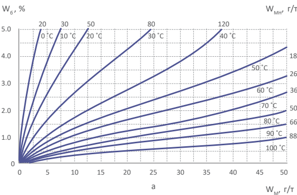
Рис.3. Кривые Ооммена: W_б – влагосодержание бумаги, %; W_м – влагосодержание масла, г/т; на полях даны насыщающие значения масла при данной температуре – W_{мн} , г/т.
