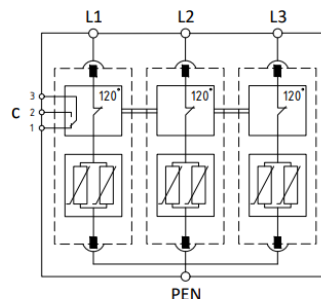
Принципиальная схема
