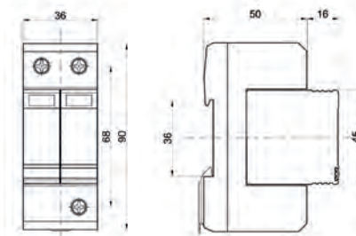
Габаритные размеры
