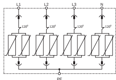
Принципиальная схема
