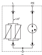
Принципиальная схема
