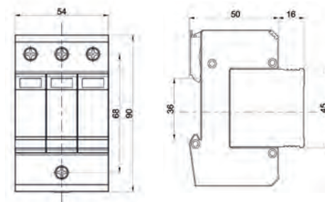
Габаритные размеры
