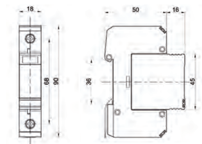
Габаритные размеры
