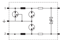
Принципиальная схема
