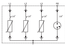
Принципиальная схема
