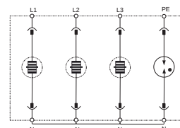
Принципиальная схема
