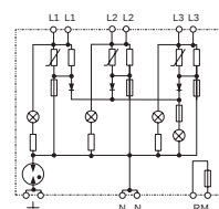
Принципиальная схема
