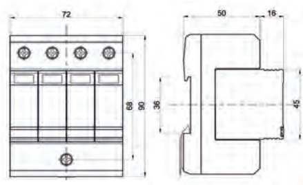
Габаритные размеры
