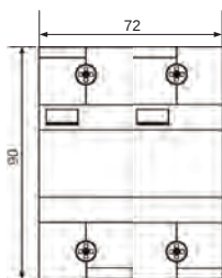
Габаритные размеры
