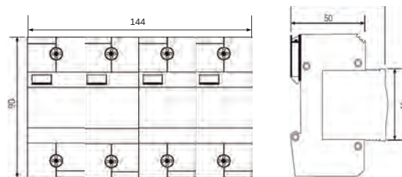
Габаритные размеры
