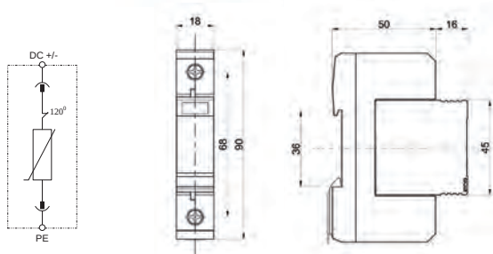
Принципиальная схема
