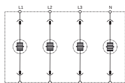
Принципиальная схема
