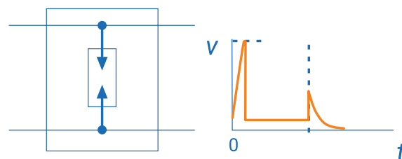
Рис. 2. Форма импульса напряжения при срабатывании УЗИП коммутирующего типа
