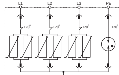
Принципиальная схема
