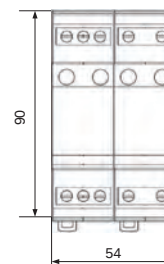
Габаритные размеры
