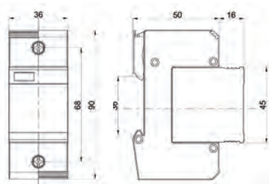
Габаритные размеры
