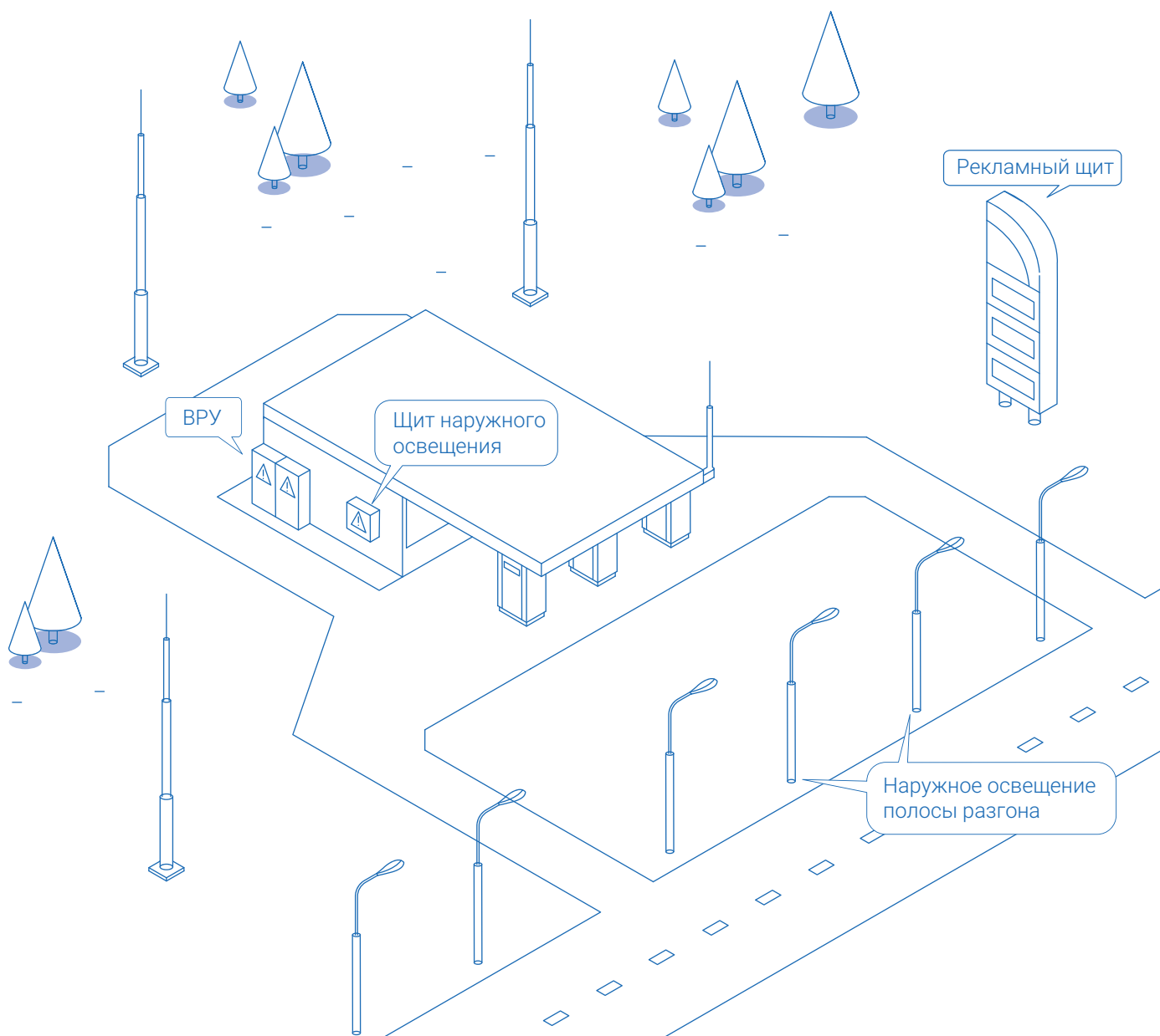
Рис. 17 – Размещение оборудования на АЗС
