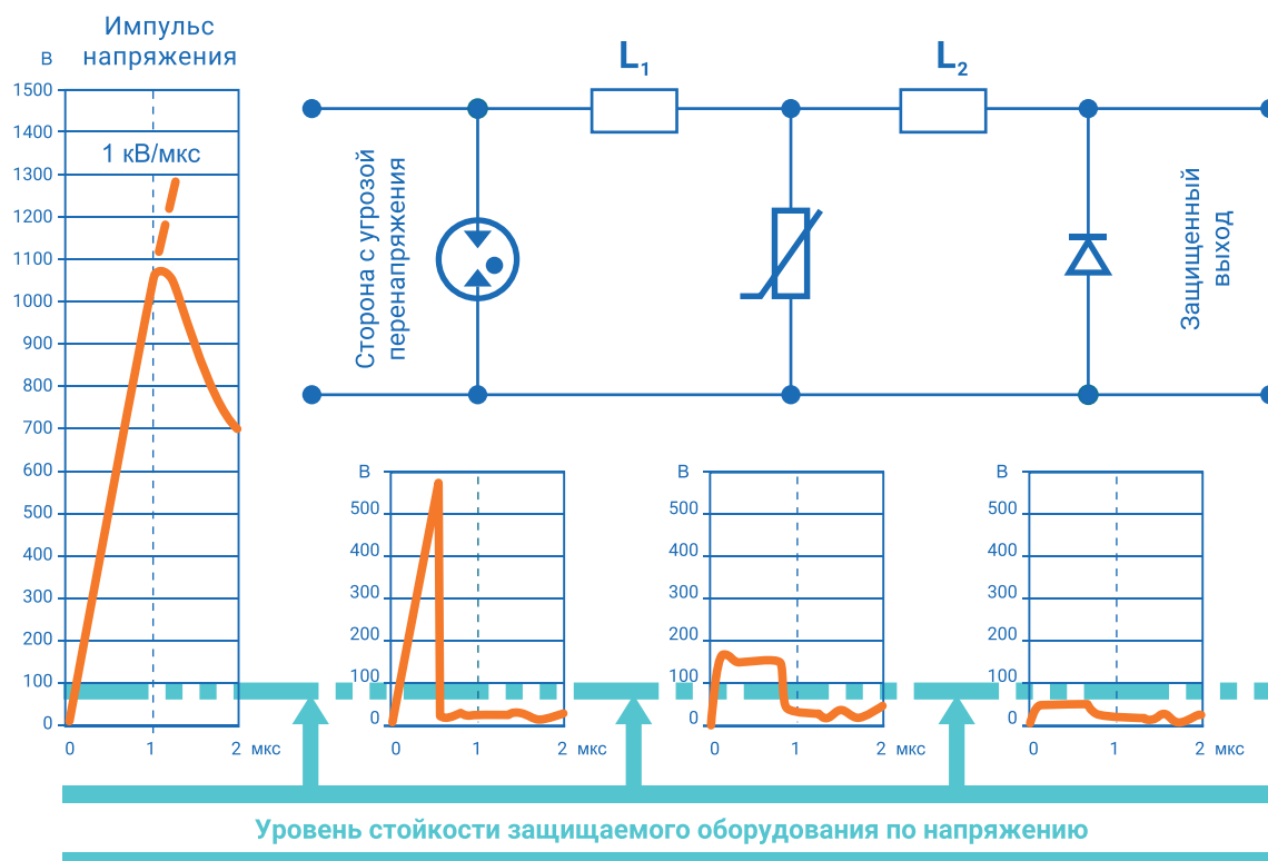
Рис. 9. Каскадная защита от перенапряжений разрядник-варистор-диод
