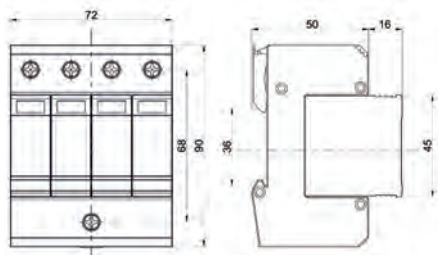
Габаритные размеры
