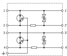
Принципиальная схема
