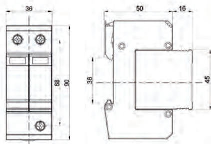
Габаритные размеры
