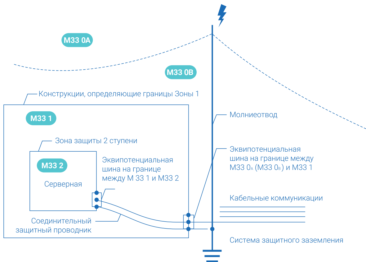
Рис 1. Применение зонной концепции молниезащиты объекта
