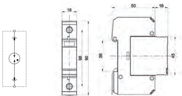
Принципиальная схема
