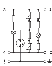
Принципиальная схема
