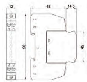
Габаритные размеры
