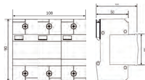
Габаритные размеры
