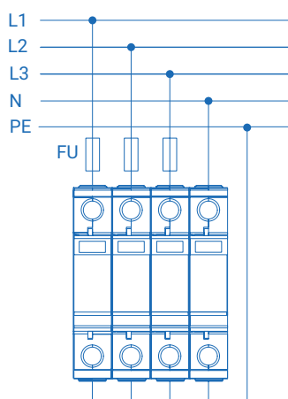
Комплект УЗИП
