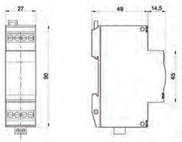
Габаритные размеры
