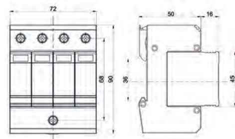
Габаритные размеры
