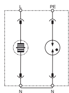
Принципиальная схема
