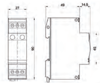
Габаритные размеры
