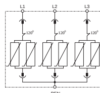
Принципиальная схема
