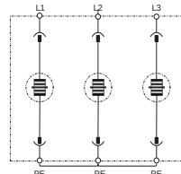
Принципиальная схема
