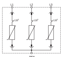
Принципиальная схема
