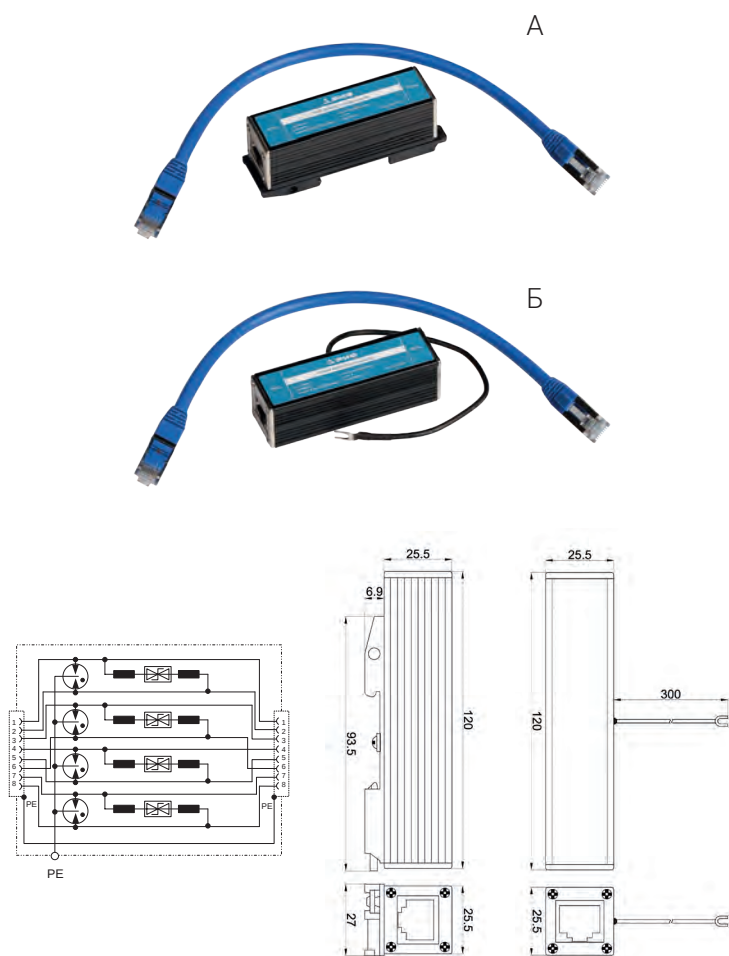
Принципиальная схема РИФ-И 48/0,5/10 (8)-кат6 (А) РИФ-И 48/0,5/10 (8)-кат6 (Б)
