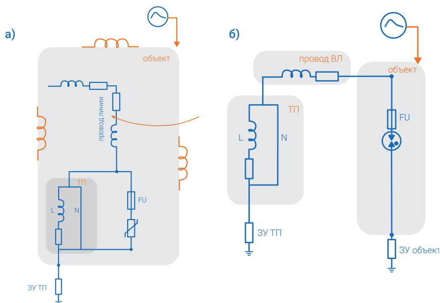
Рис. 13 – Схемы замещения для оценки токов через УЗИП при наличии у объекта системы молниезащиты: а) отходящих линий нет; б) от объекта отходит линия 0,4 кВ
