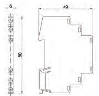
Габаритные размеры
