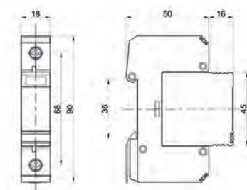
Габаритные размеры
