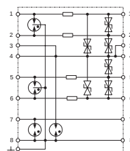
Принципиальная схема
