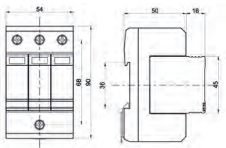
Габаритные размеры
