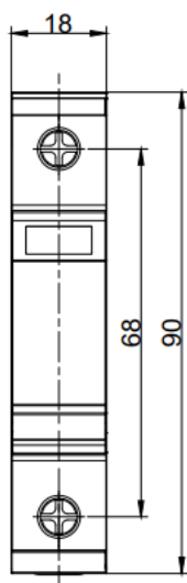
Габаритные размеры
