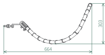
Габаритные размеры РДИП-10
