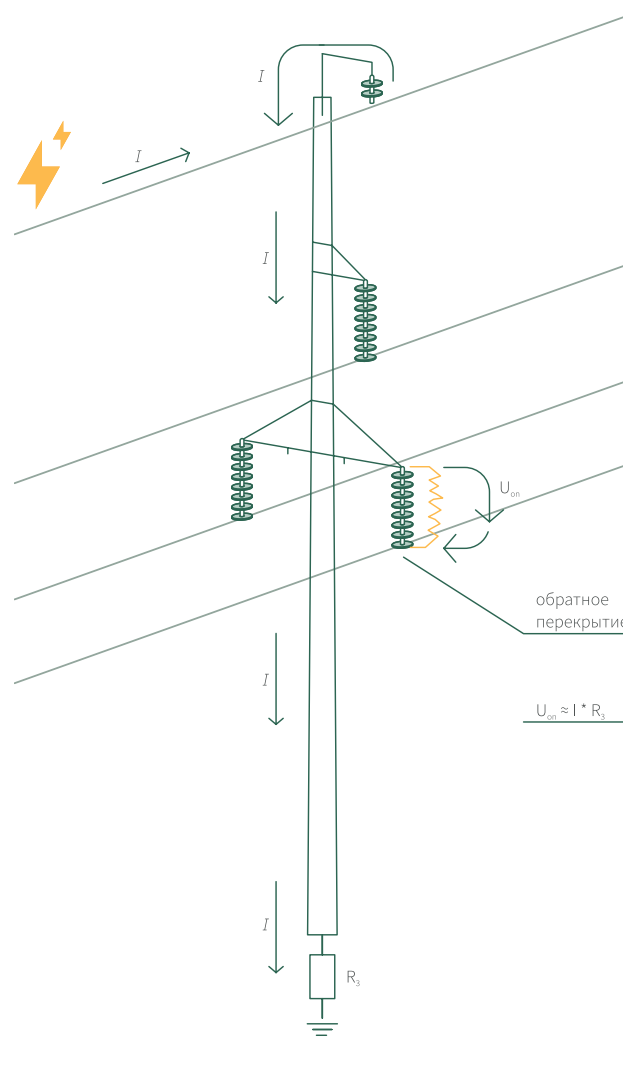
Схема 9. «Обратное» перекрытие изоляции
