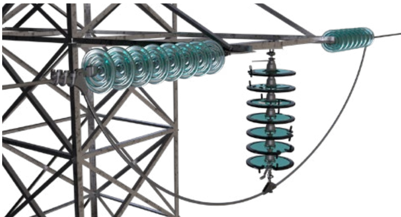
Рис. 26. Установка гирлянды ГИРМК-110 на анкерно-угловой опоре
