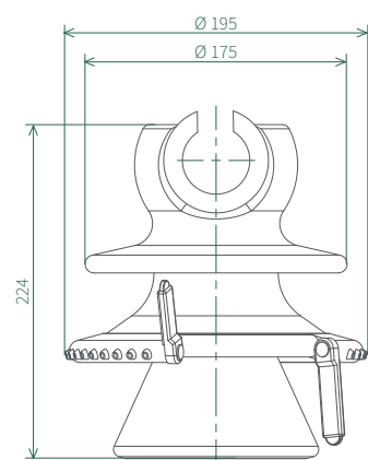
Габаритные размеры ИРШФМК-10(20)
